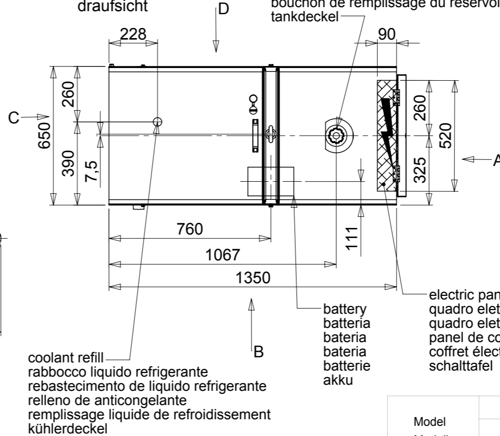
top view vista superiore vista superior vista superior vue de dessus draufsicht
