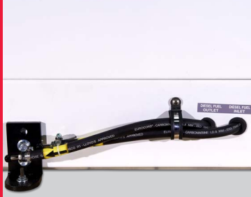
Ingresso e uscita gasolio
