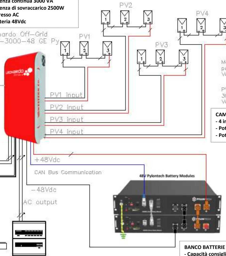
Fig.4 Schema di collegamento
