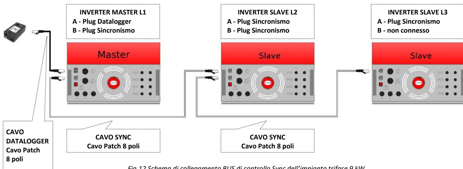
Fig.12 Schema di collegamento BUS di controllo Sync dell'impianto trifase 9 kW
