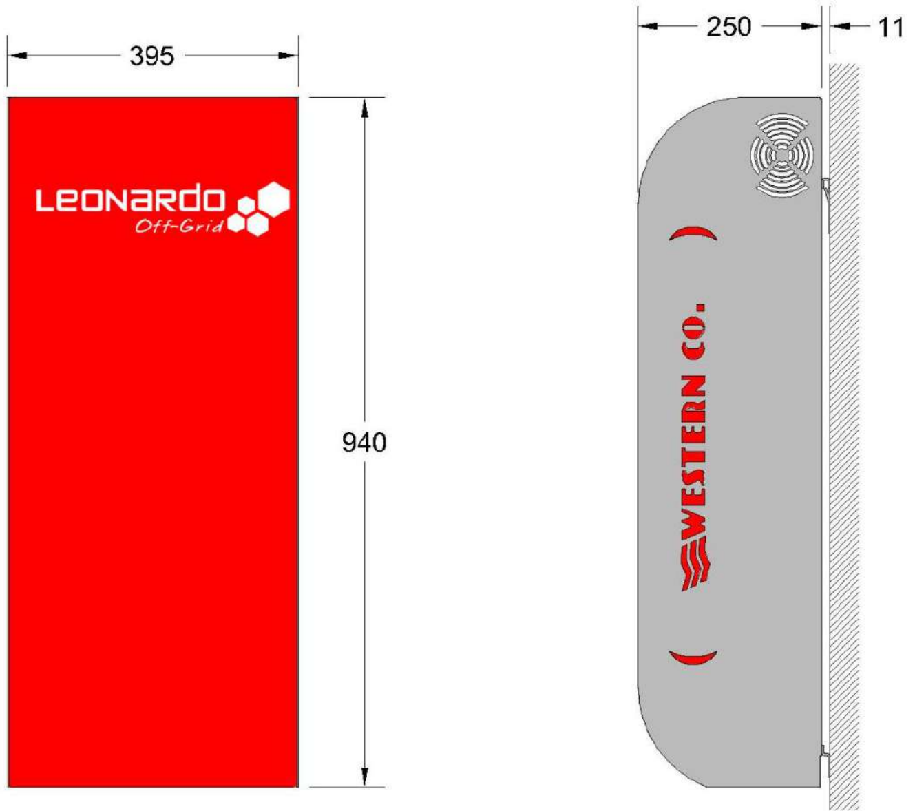
Fig.16 Caratteristiche meccaniche
