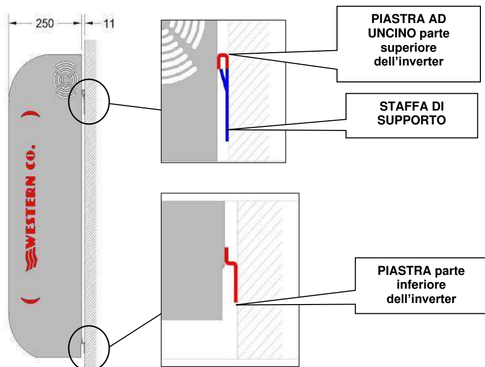
Fig.10 Montaggio a parete
