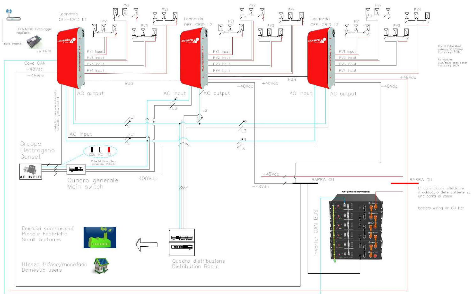
Fig.13 Schema Unifilare dell'impianto trifase 9Kw
