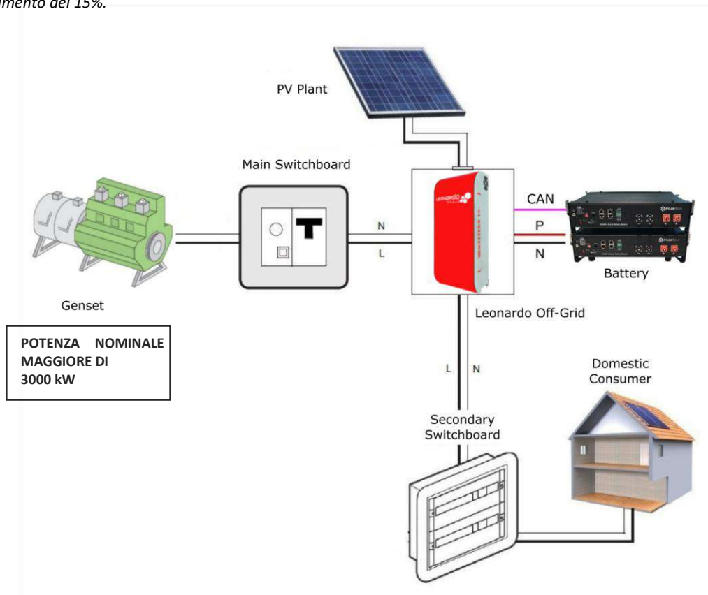
Fig.2 Schema di principio
