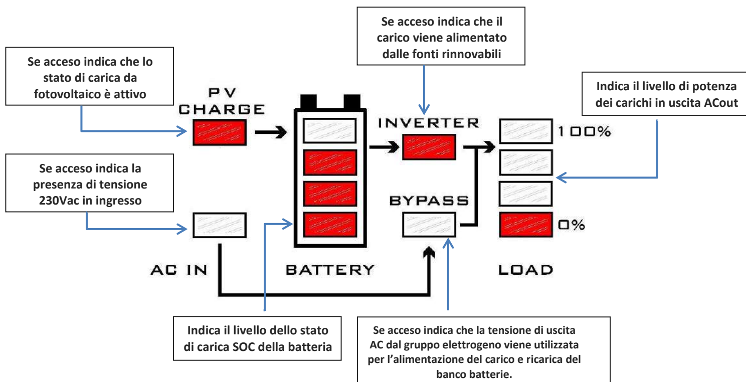
Fig.8 Segnalazione Energy Manager
