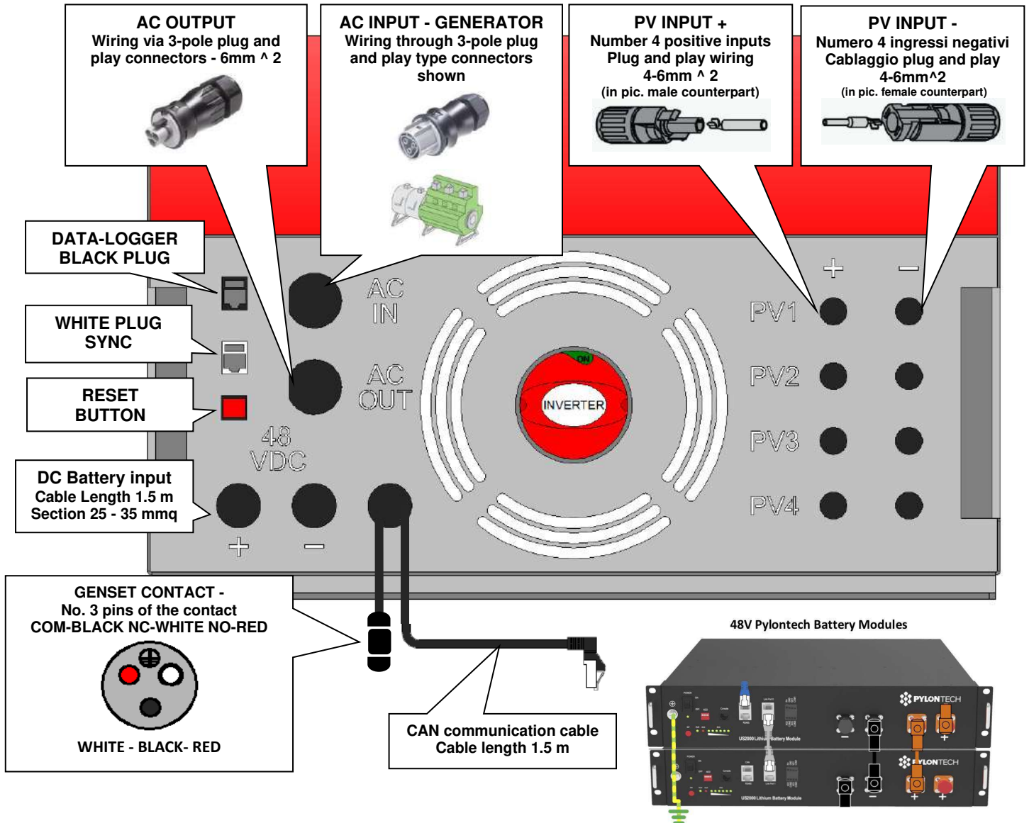
Pic.11 Wiring
