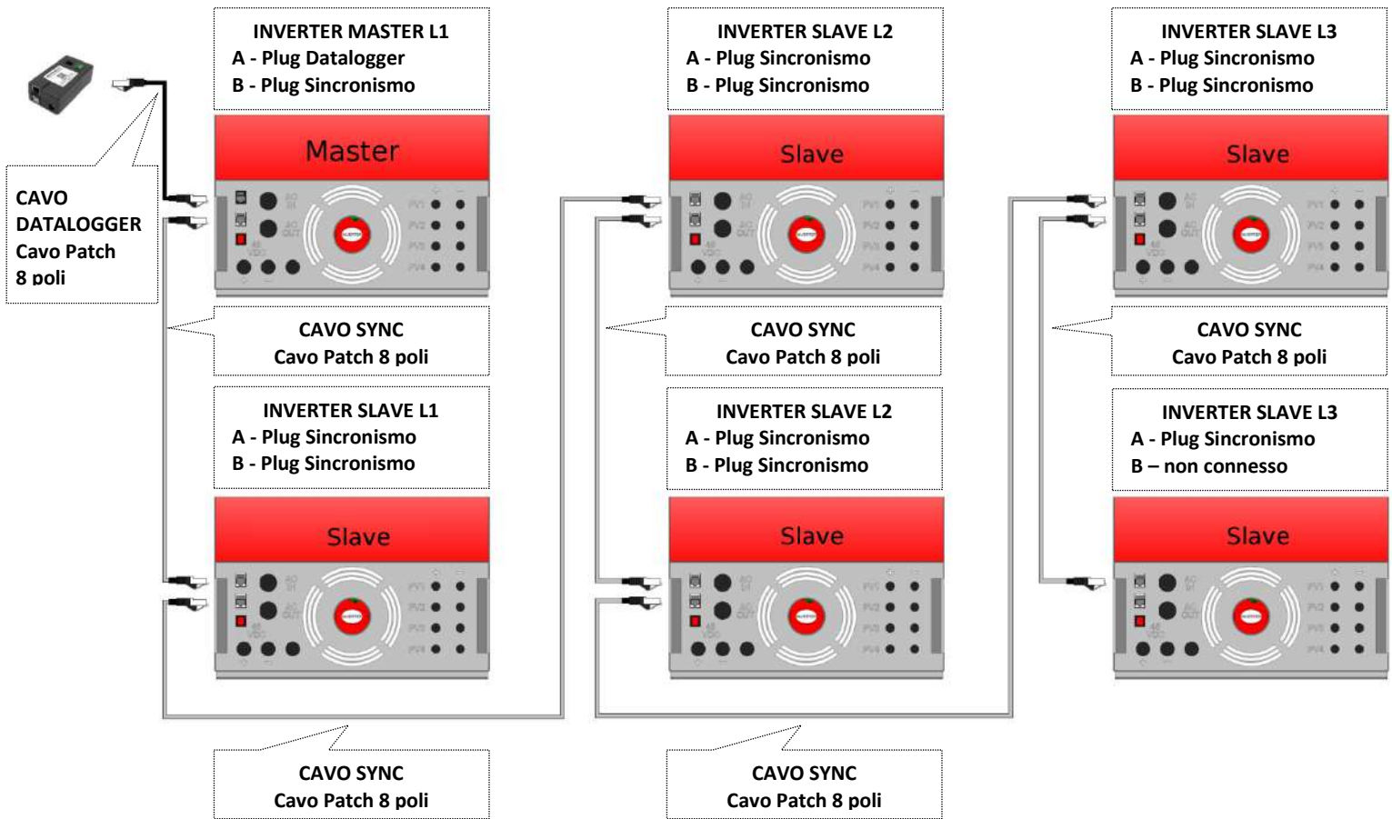
Fig.14 Schema di collegamento BUS di controllo Sync dell'impianto trifase 18 kW
