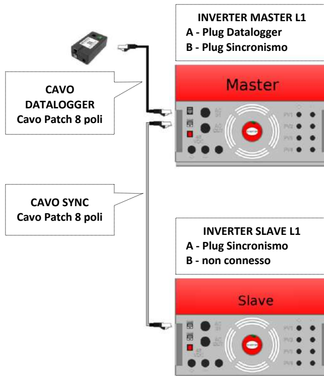
Fig.15 Schema di collegamento BUS di controllo Sync dell'impianto parallelo 6 kW
