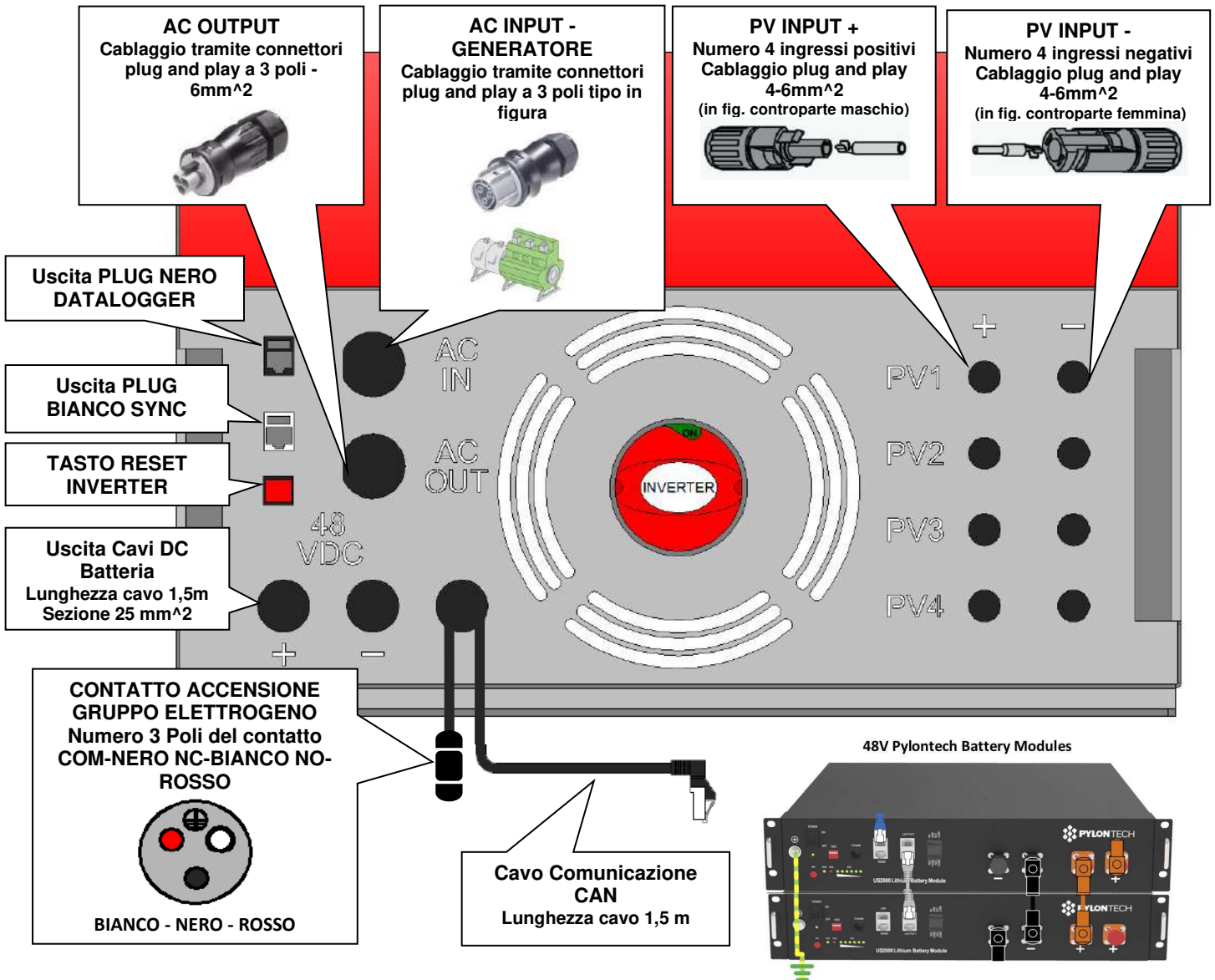
Fig.11 Cablaggio
