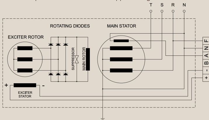
FIG. 1: Schema per regolatore di tensione tipo S125 su alternatore brushless.
